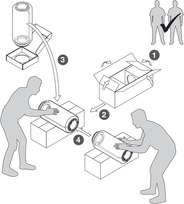
Fig. 6 2-3-4 Cylinders
