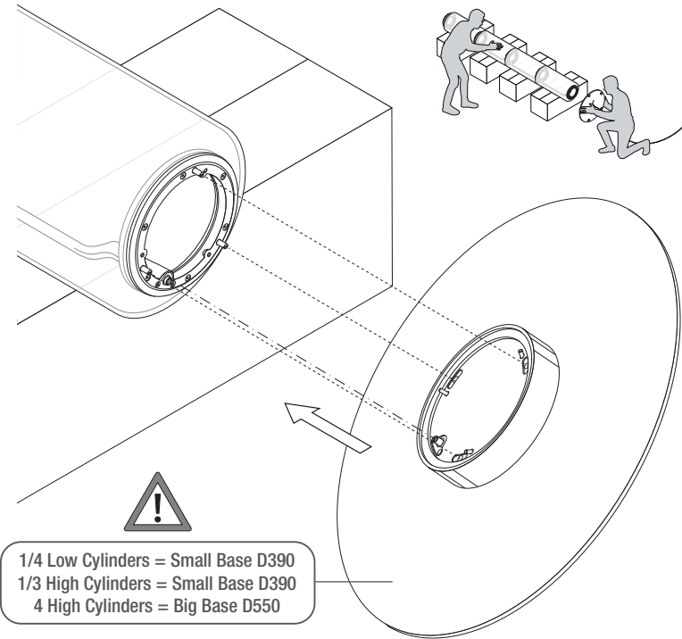
Fig. 8 2-3-4 Cylinders
