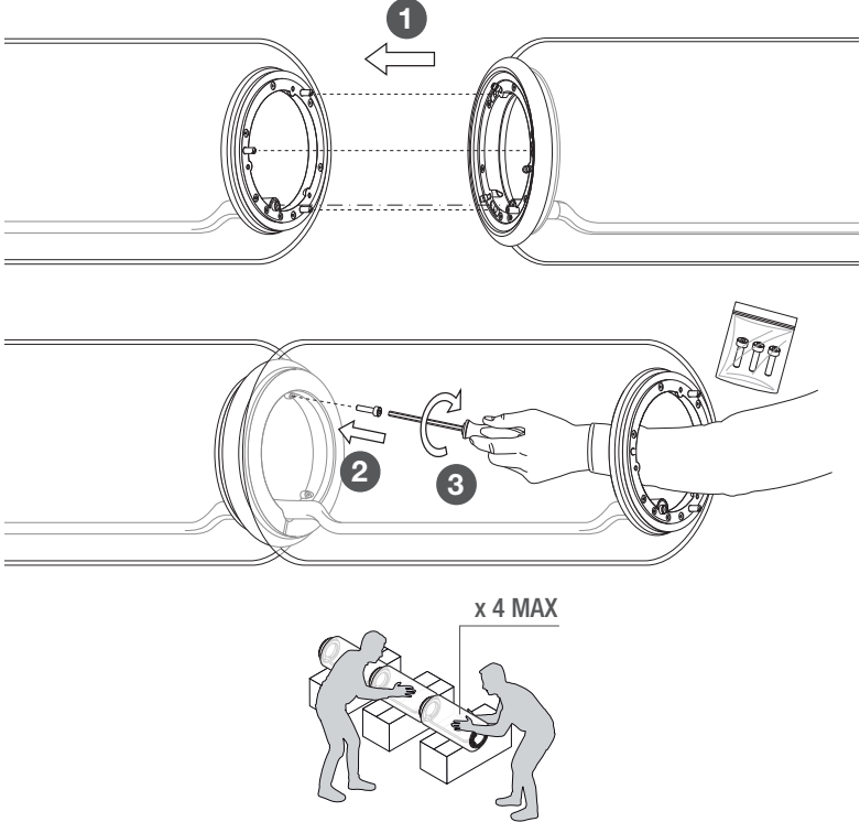
Fig. 7 2-3-4 Cylinders
